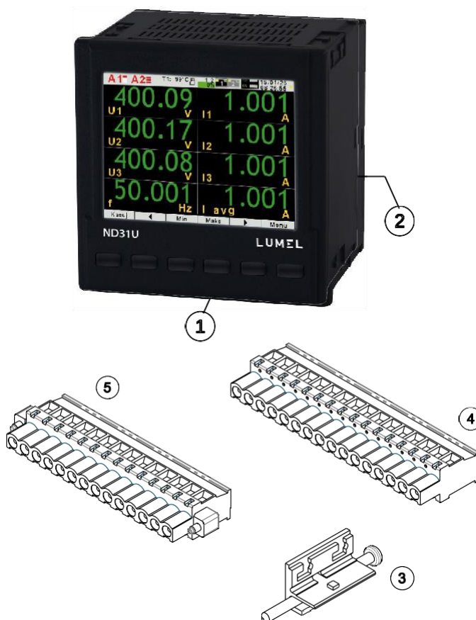
Fig. 1. Meter set
